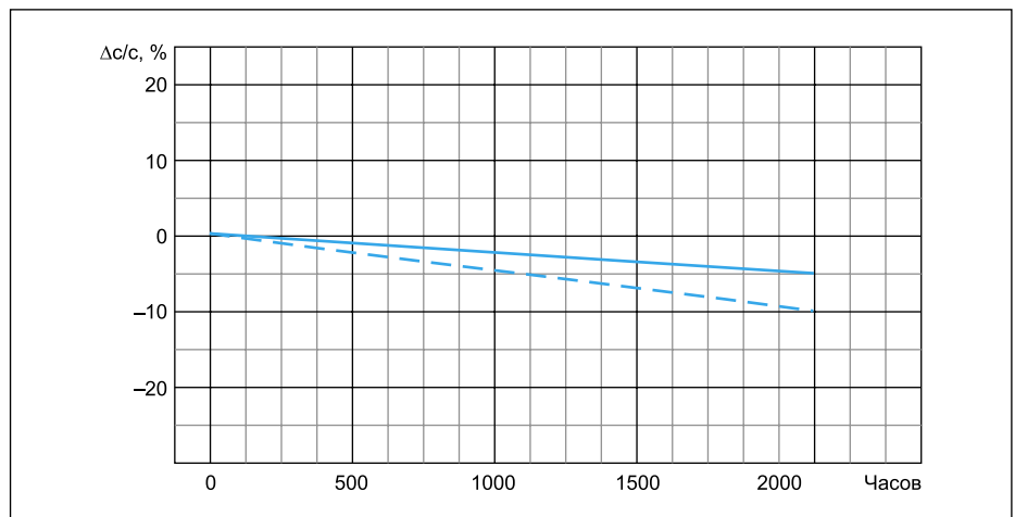
Рис. 6. Зависимость емкости конденсаторов серии GM от наработки
